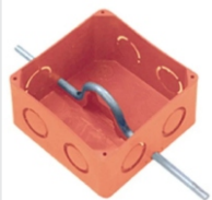
Orange Fan Box 104 x 104 x 52
